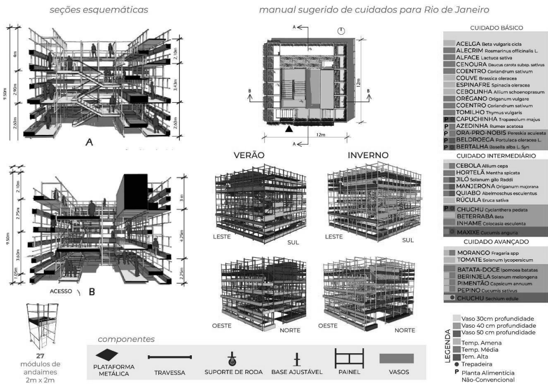
Figure 2. Esquemas arquitetônicos e de plantio para cada fachada do dispositivo Trama. Autora: Rebeca Waltenberg.
